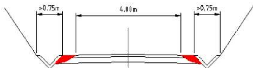
Secció de vial en desmunt
