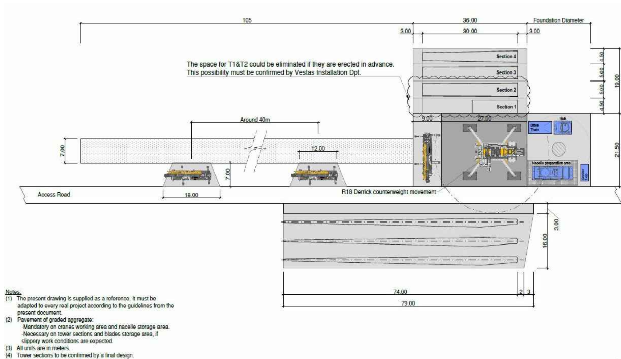
PLATAFORMA DE MUNTATGE TIPUS (cotes en metres)
