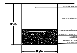
RASA PER TRES O MES CIRCUITS
