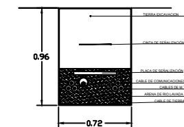
RASA PER DOS CIRCUITS
