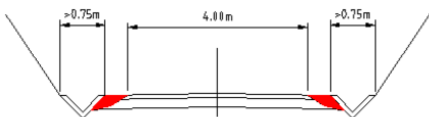
Secció de vial en desmunt
