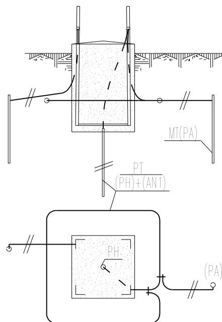
Esquema 1.14 - Toma de tierra en zona no frecuentada agrícola (A)
