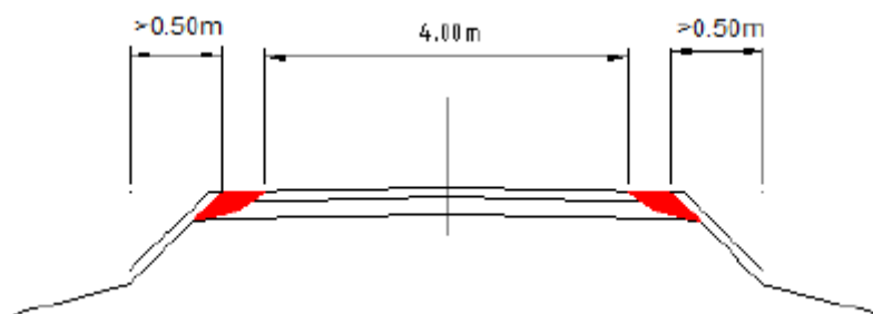
Secció de vial en terraplens
