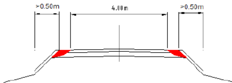
Secció de vial en terraplens
