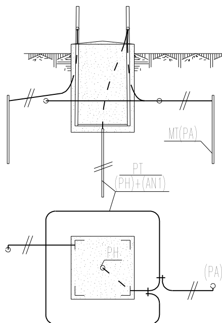
Esquema 1.14 - Toma de tierra en zona no frecuentada agrícola (A)
